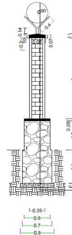
Section A-A
